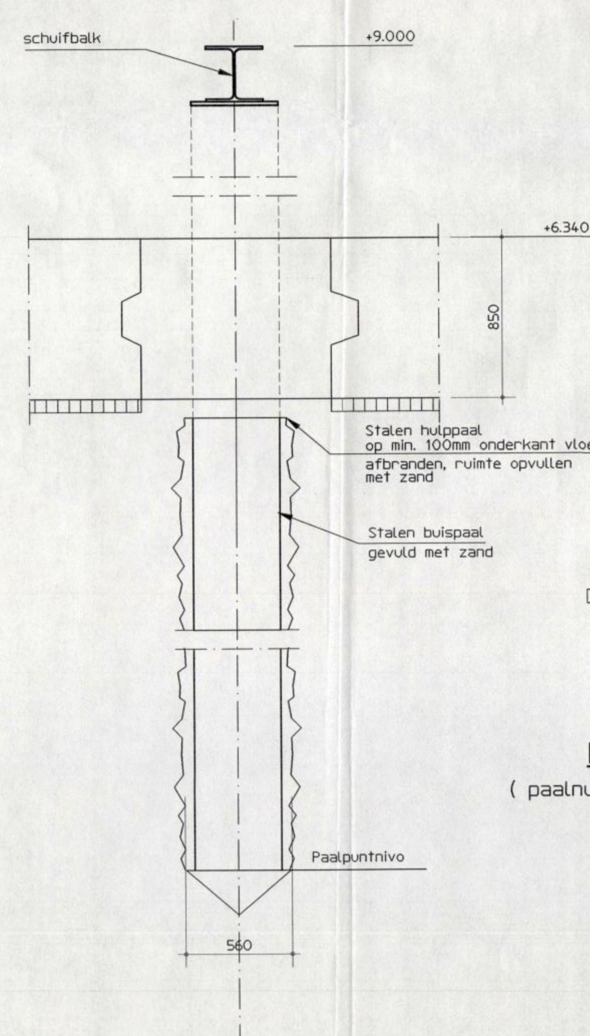
Detail Tubexpaal 1:20 In definitieve situatie
