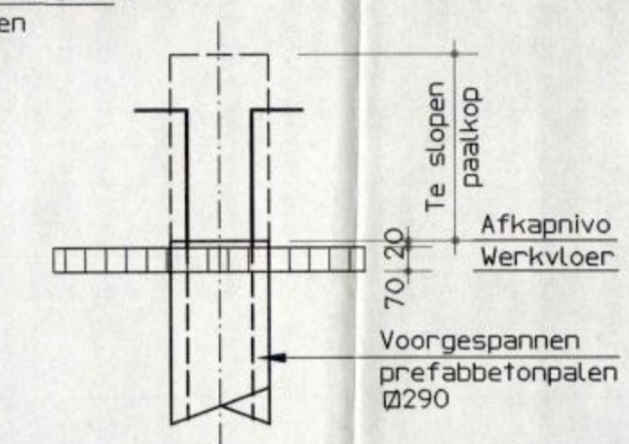
Detail paalkop 1:20 (paalnummer 1 t/m 44 en 59 t/m 72)
